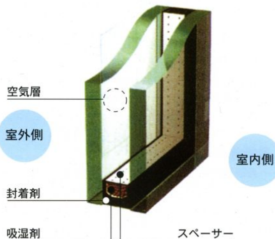
エコガラスの断面図
